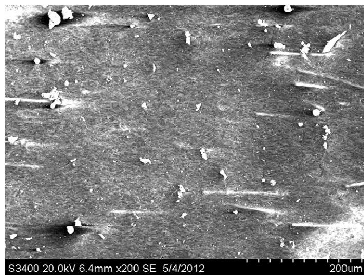
b. SEM, USED-CM68
