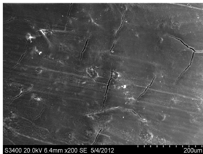
a. SEM, NEW-CM68
